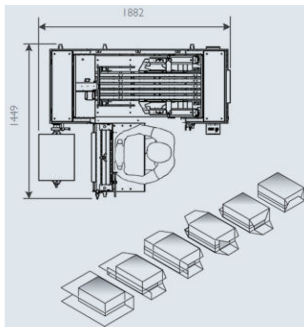
Slika 3. Princip rada mašine
