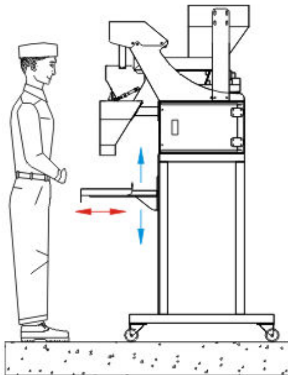
Jedna merna glava sa jednim vibracionim kanalom
