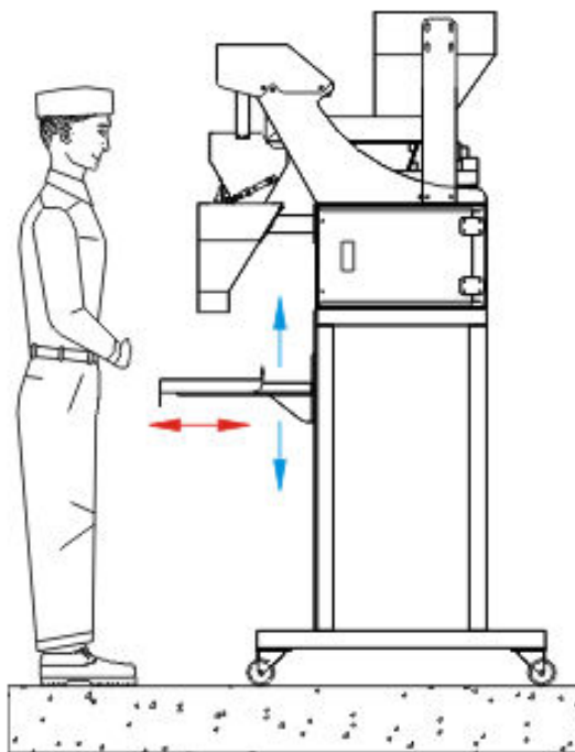
Jedna merna glava sa dva vibraciona kanala
