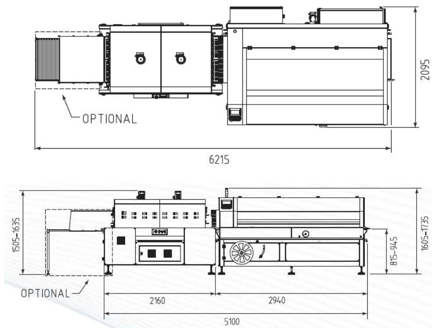
Slika 3. Dimenzije mašine HS800
