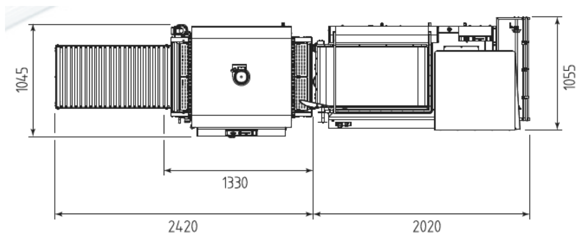
Slika 8. Dimenzije mašine FP870A
